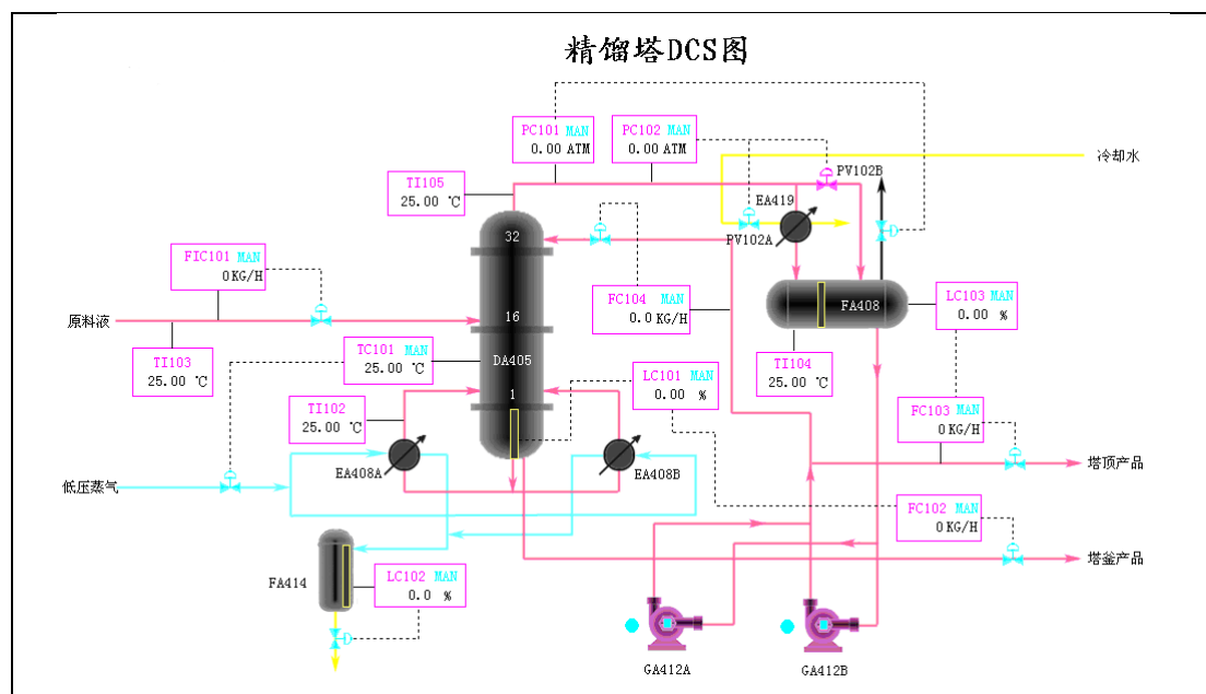
图 2-13 精馏 DCS 图
