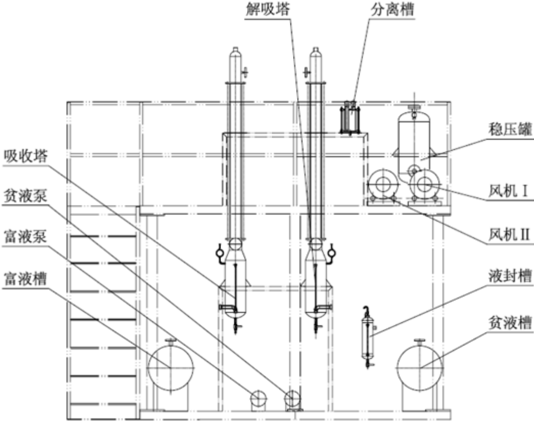
图 5-2 吸收-解吸操作立面图
